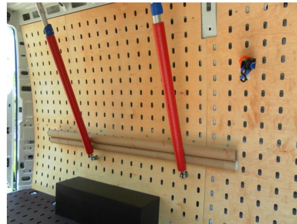
Durch die Verbindung Wand zu Decke können lange oder runde Teile unverrollbar transportiert werden. Der Fahrzeugboden bleibt frei für zusätzliches Ladegut.
